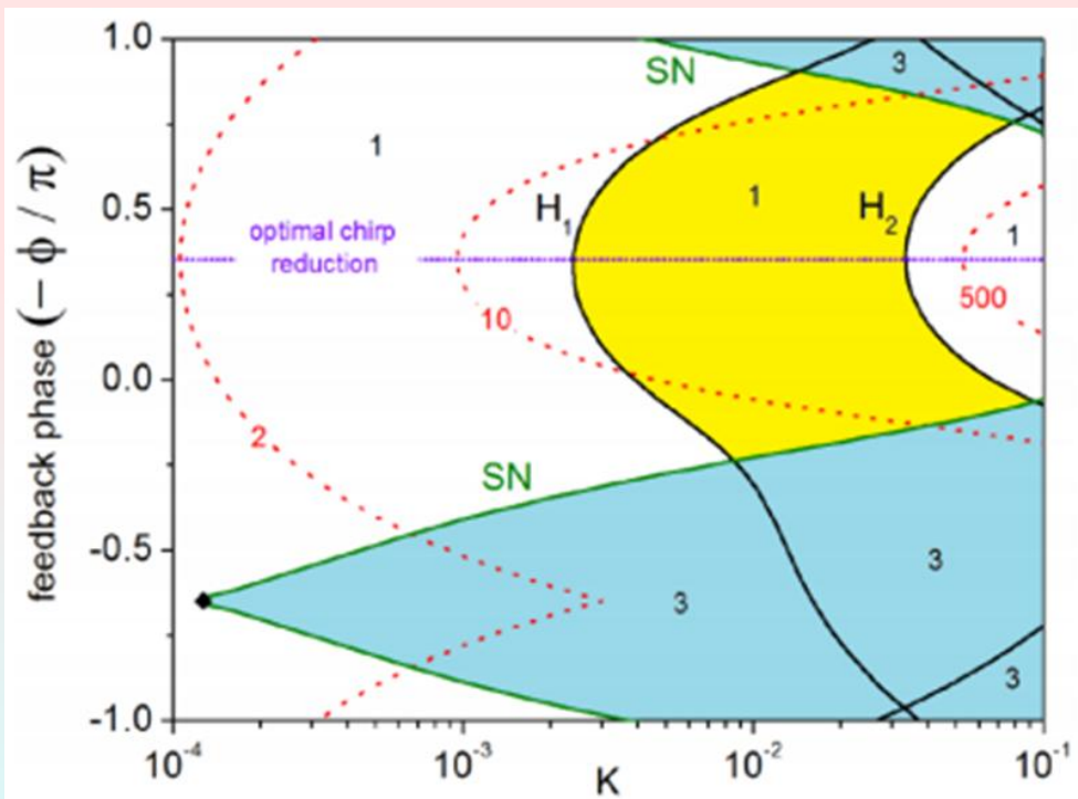
Diagrama bifurcațiilor din sistem
