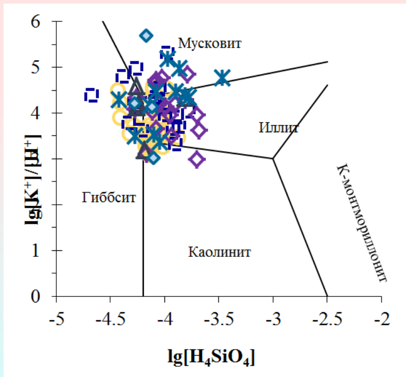
Diagramele echilibrului geochimic a apelor freatice cu mineralele alumo-silicate
